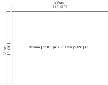
Cutout Dimensions
